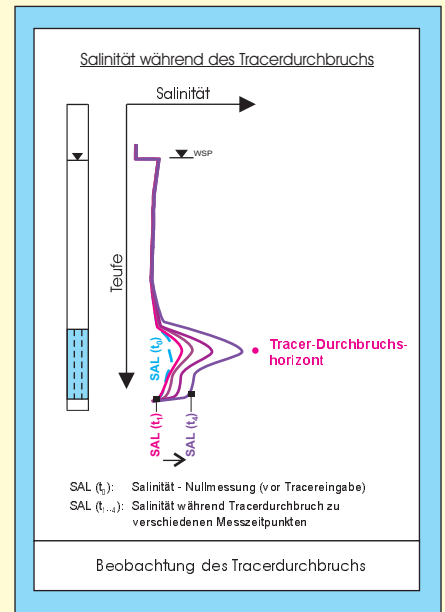
Registrierung des Tracerdurchbruchs in einer Empfangsmessstelle bei Mehr-Bohrloch-Versuchen (Prinzipbild)
