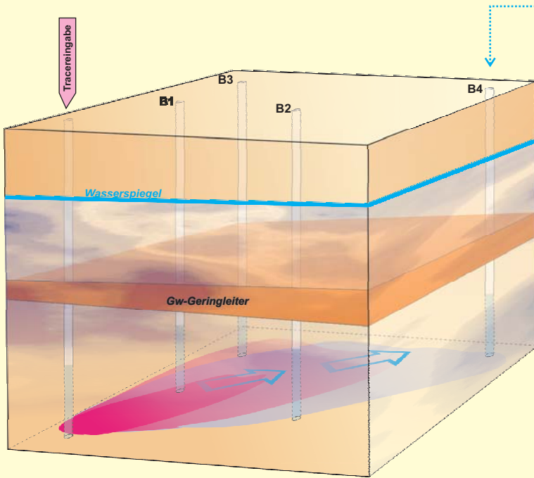
Registrierung des Tracerdurchbruchs in einer Empfangsmessstelle bei Mehr-Bohrloch-Versuchen (Prinzipbild)
