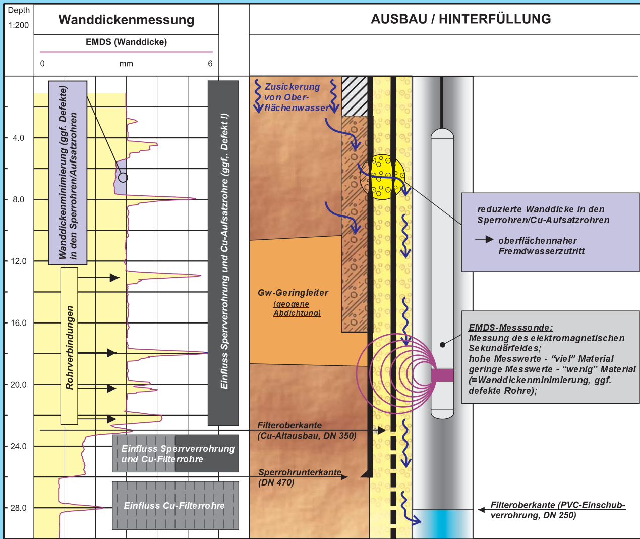
Prinzip und Beispiel für den Einsatz einer elektromagnetischen Wanddickenmessung (EMDS)
